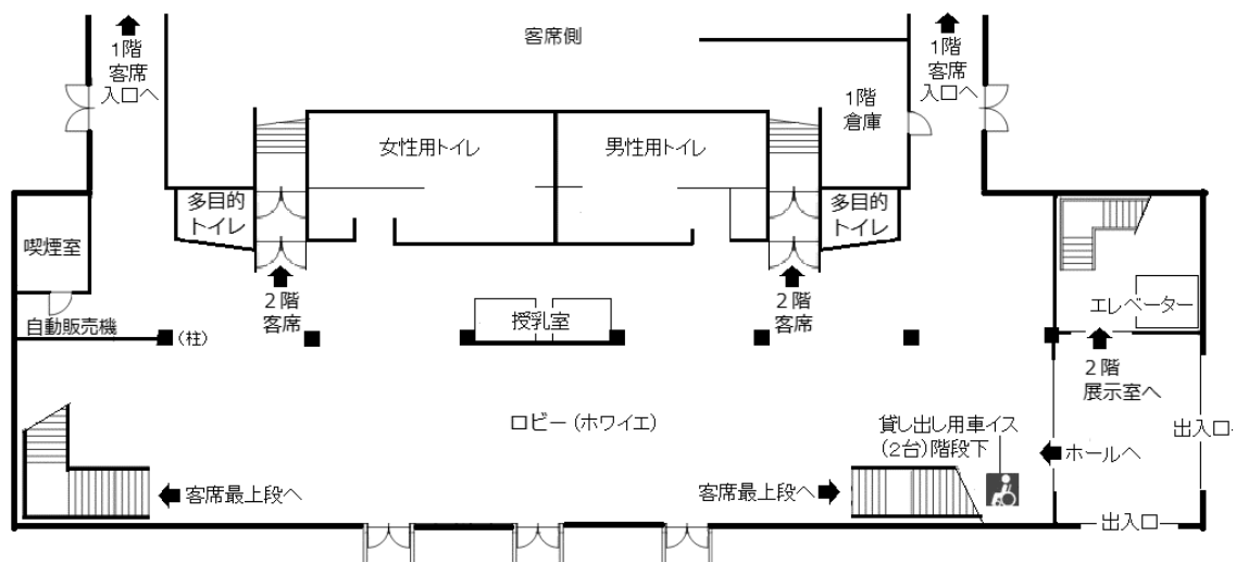
ロビー（ホワイエ）配置図
